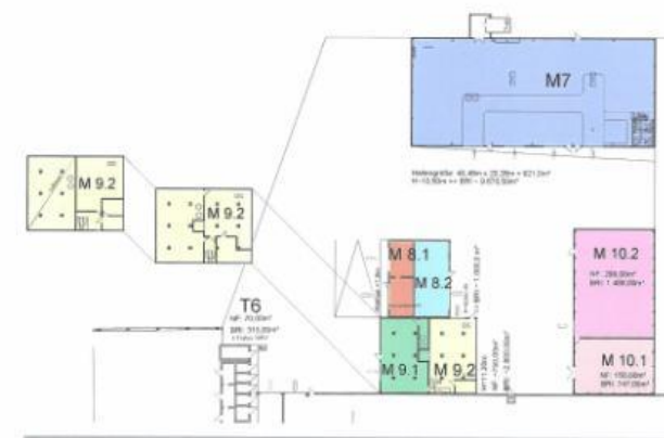
Plan M7-M10 (Handwerkerhof)
